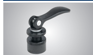
Elemento de paragem e fixação Ø30 mm (Art.No. 5198150)
