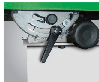
Mesa inclinável de 0 a 45°
