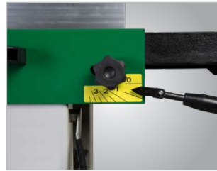
Ajuste da remoção de material através de alavanca de controlo
