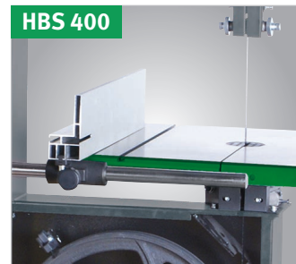
Mesa inclinável de 0 a 45°
