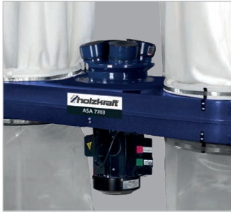
Unidade de extração rotativa em 180° permite a orientação da sucção por baixo ou por cima (Fig. mostra ASA 7703)
