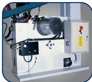
Inclinação da mesa através de cremalheira e chave estrela / delta automática
