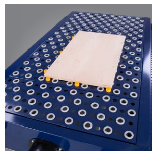
Batentes inseríveis para fixar a peça
