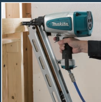
AN924 - Chiodatrice
