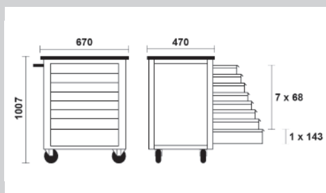
Medidas externas
