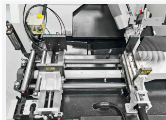
Alimentação de material através de fuso de esferas
