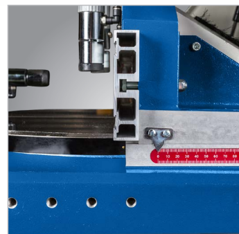
Batente continuamente ajustável
