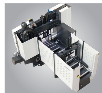
Alimentação de material com 2000 mm de comprimento
