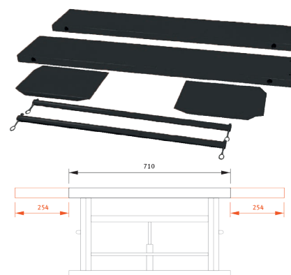
MHB 680 com extensão lateral
