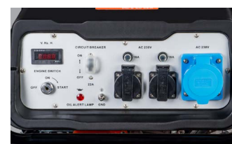
Modelo do painel comando PG-E 90 SEA
